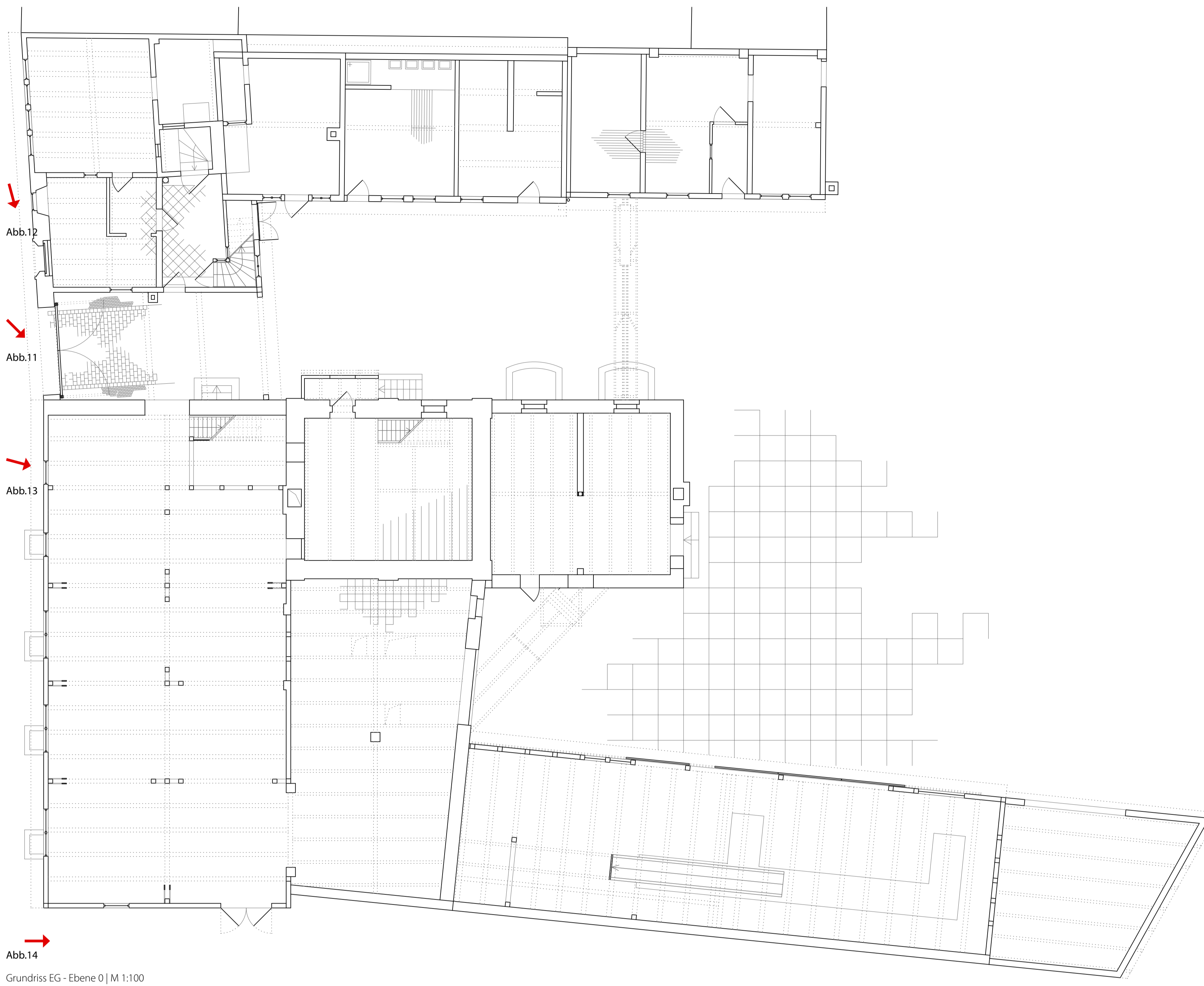
Grundriss EG - Ebene 0 | M 1:100
