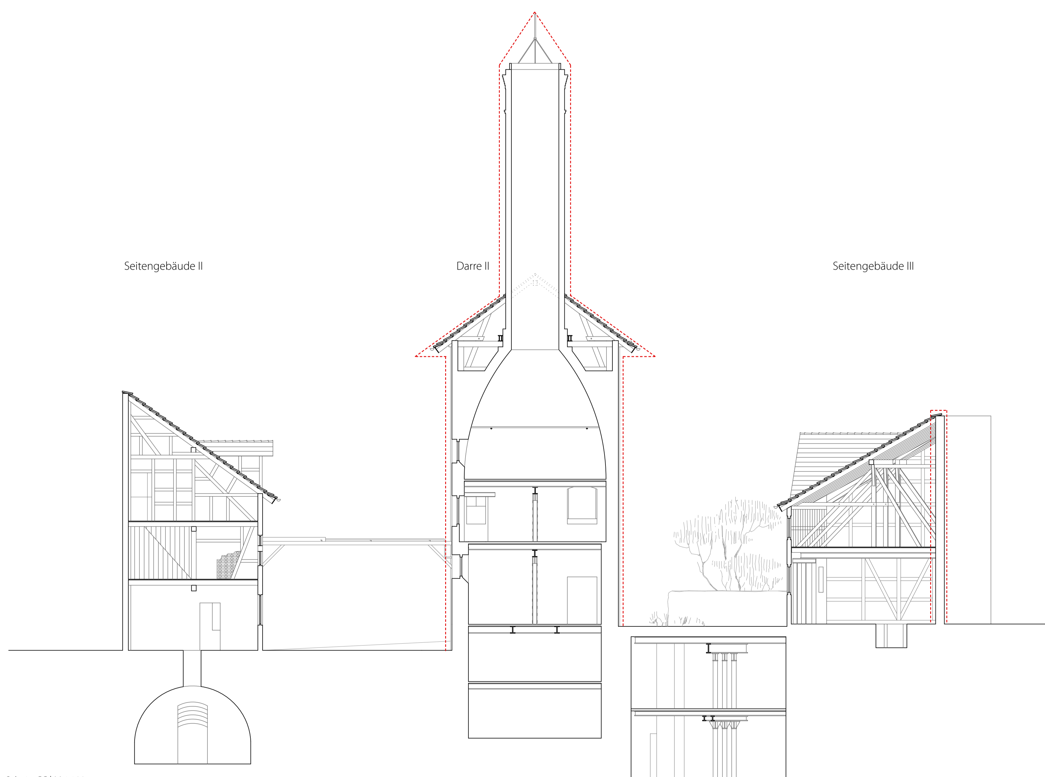
Schnitt CC | M 1:100
